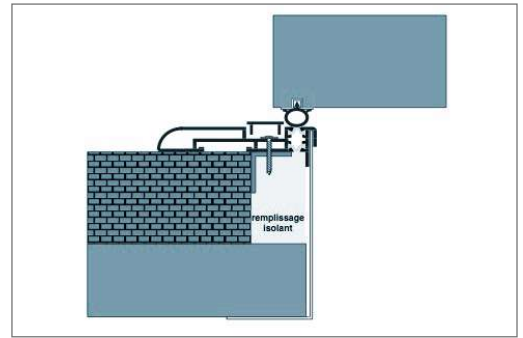
Montage sur maçonnerie
